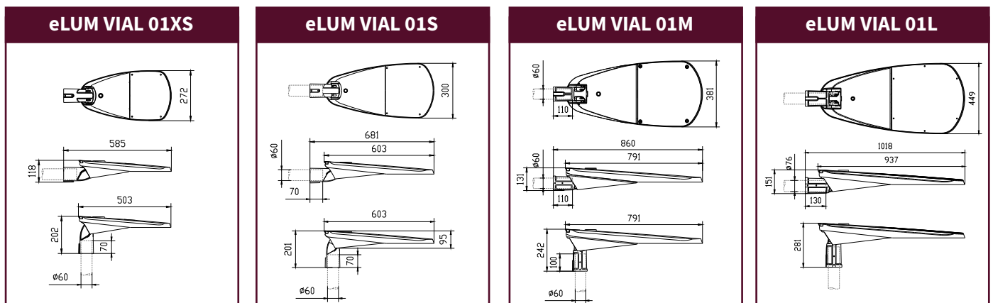
Dimensiones en mm
